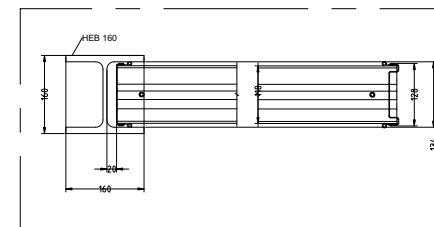
1:5 Schemat montażowy
