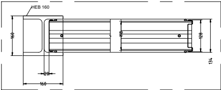
1:5 panel BUDAN - montaż
