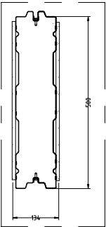
1:5 Panel BUDAN przekrój
