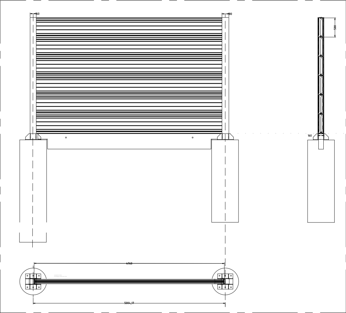
1:20 Widok ogólny
